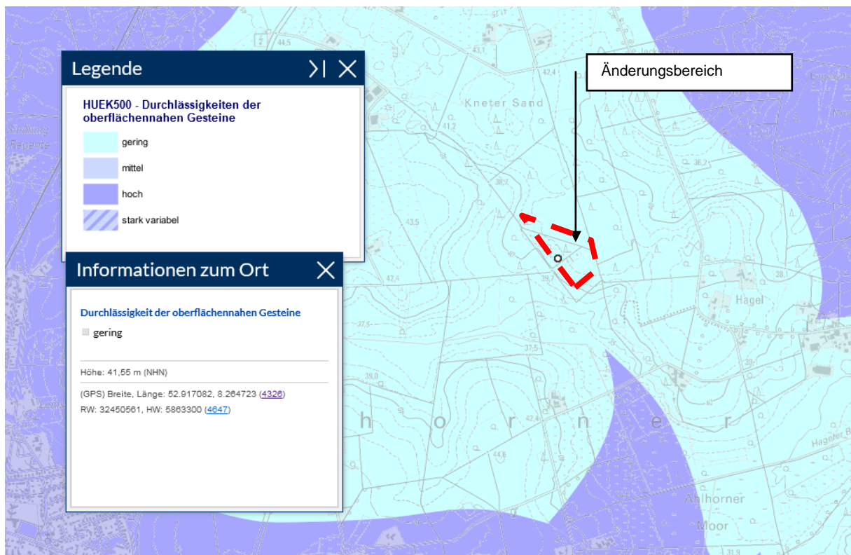
Abbildung 8: Durchlässigkeit der oberflächennahen Gesteine, unmaßstäblich (LBEG 2024)
