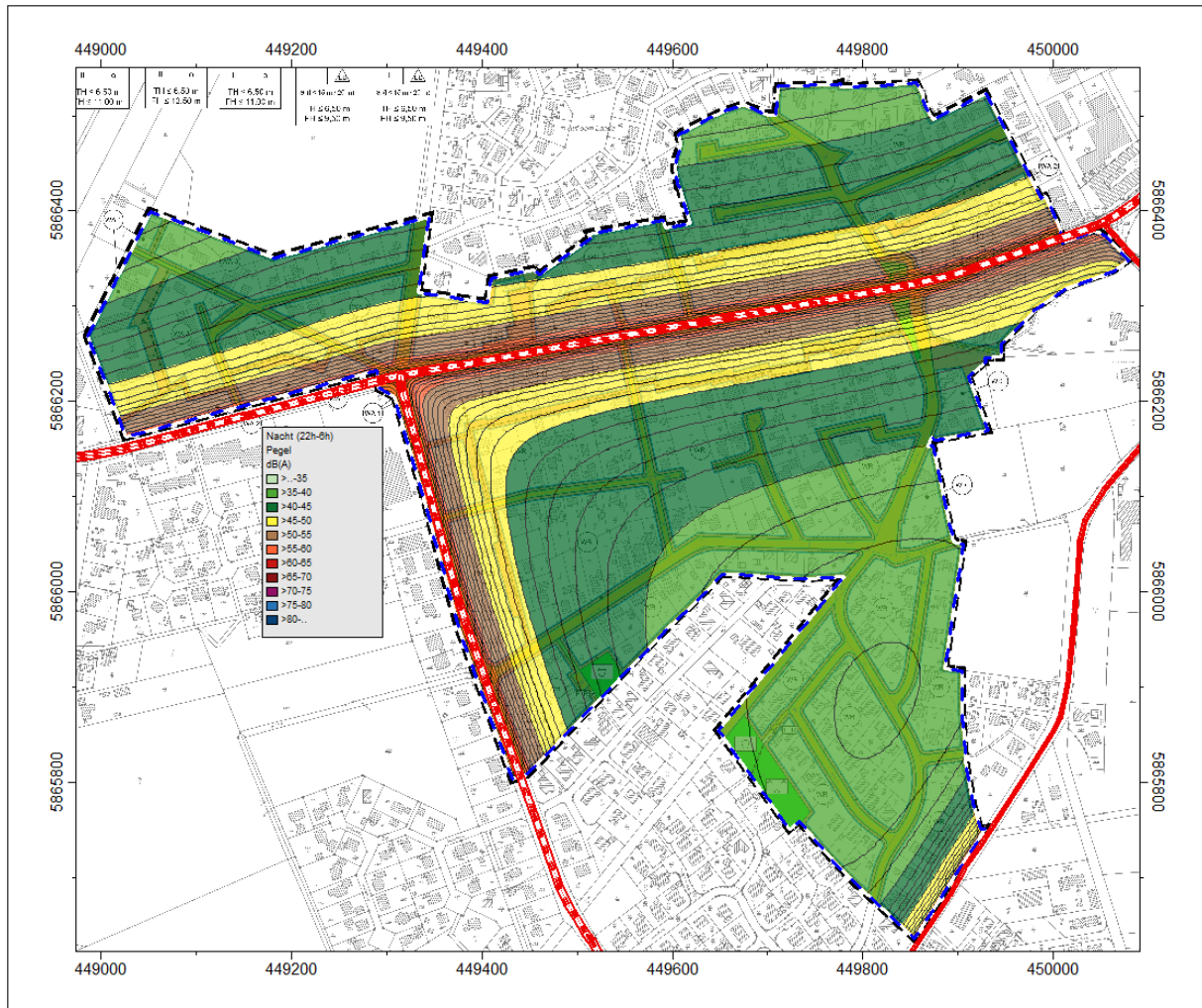
Abbildung B2: Beurteilungspegel „Straße“ nachts, OG (4,8 m über Grund).
