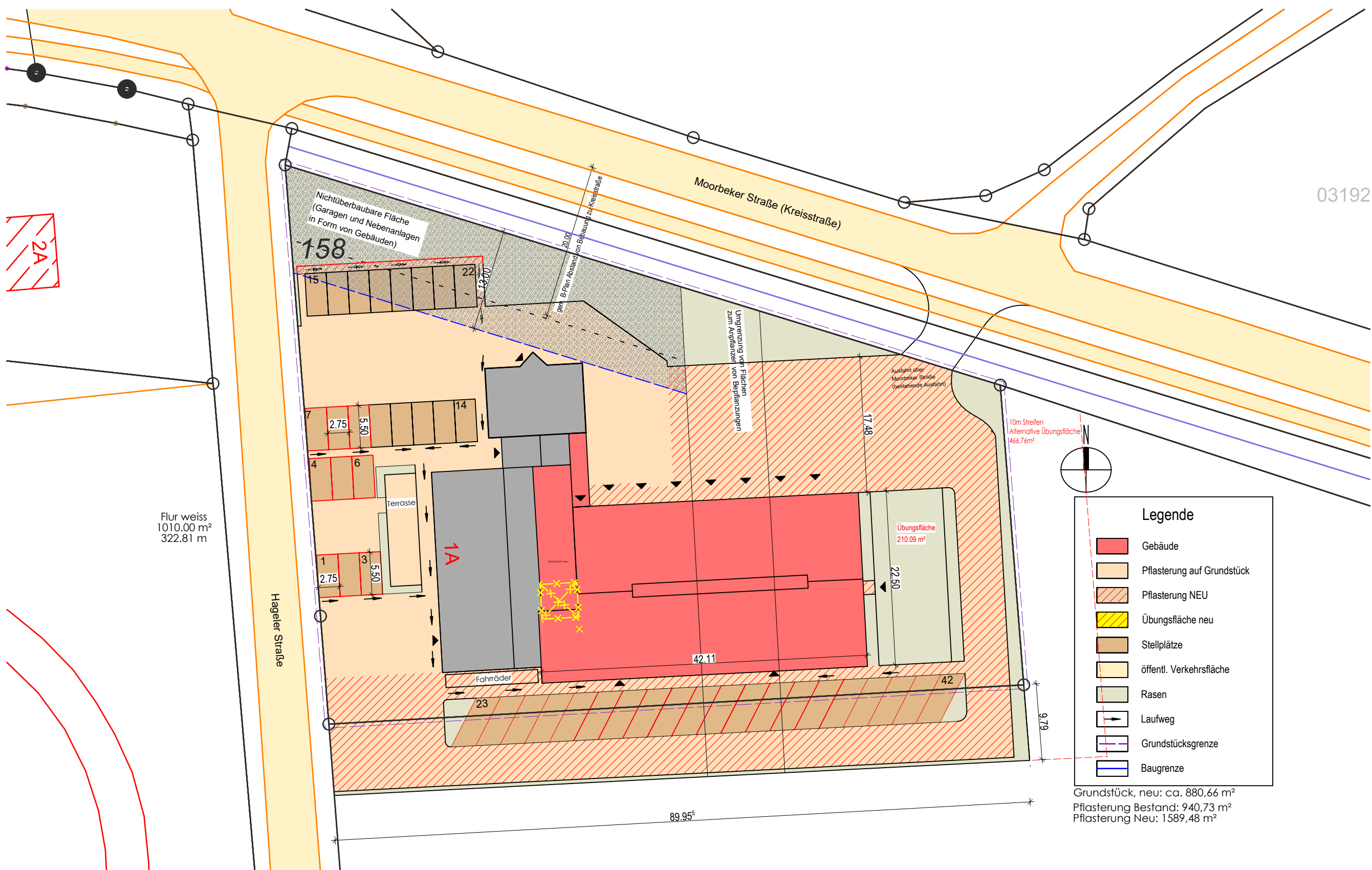
Lageplan - Variante 5
